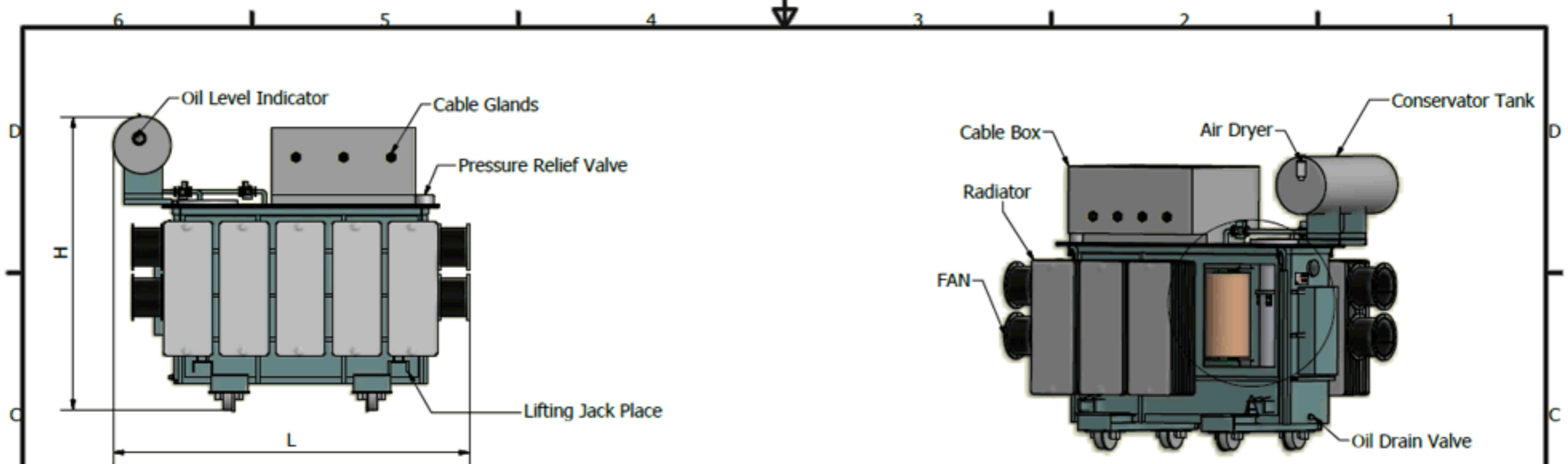
A ( 1 : 20 )
